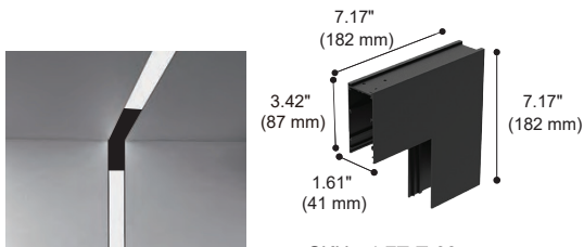
SKU : LFT-T-03 Type : 7 Type vertical corner
