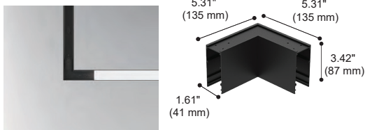
SKU : LFT-T-02 Type : L Type horizontal connector
