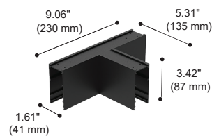
SKU : LFT-T-04 Type : T Type horizontal connector
