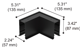
SKU : LFT-F-02 Type : L Type horizontal connector
