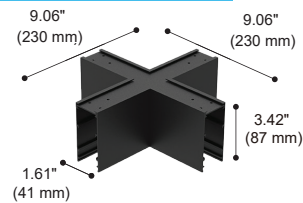
SKU : LFT-T-05 Type : X Type horizontal connector
